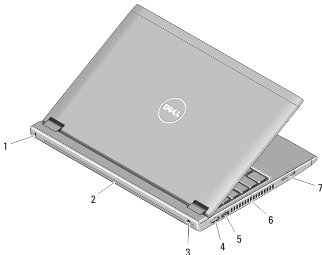
圖 2. 後視圖
