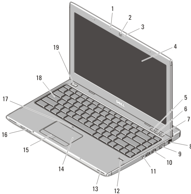
圖 1. 前視圖
